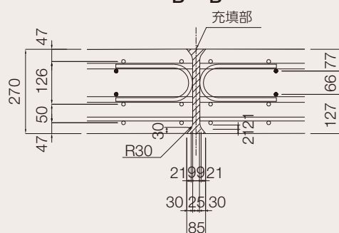
床版支点部 B-B
