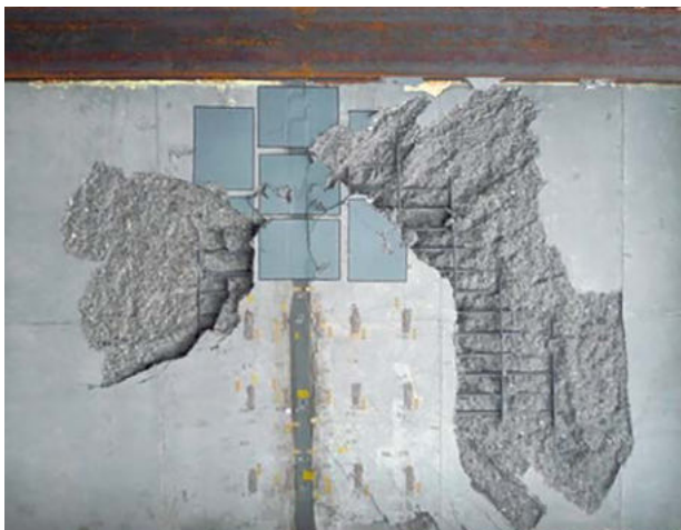
床版下面の破壊状況
